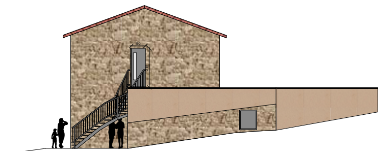
Façade Est - PRO Echelle: 1:100
